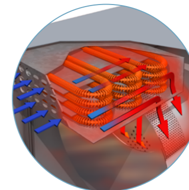
ELEKTRISCH BEHEIZT
